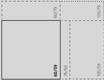
Dimensiones del cristal con quemador Prestige (modelos GP)
